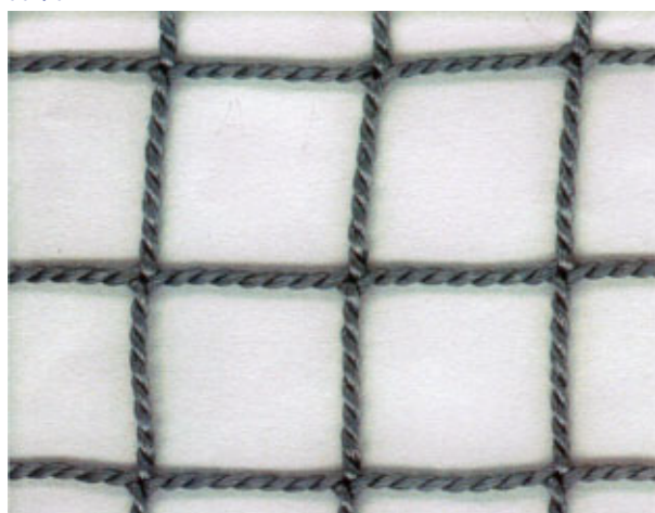
ポリエチレン 無結節網 目合 25 mm シルバー (糸径 約 2.1 mm)
