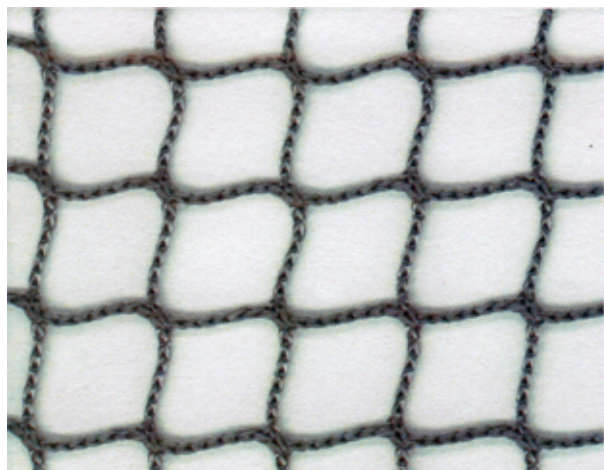
ポリエステル ラッセル網 目合 15 mm グレー (糸径 約 1.5 mm 防炎加工品)
